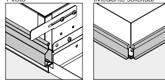
Aplicación en techos modulares SAS 150/330 (Mediante solicitud)
