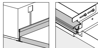
Aplicación en techos modulares de perfil en T visto
