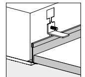
Aplicação sob tetos modulares de perfil T visível com niveladores
