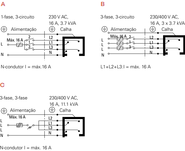
Esquema elétrico
